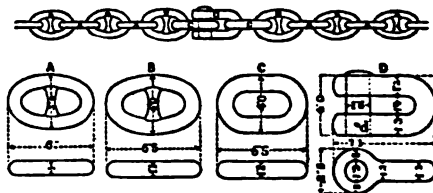
FIG. 1.—Stud-link Chain.
