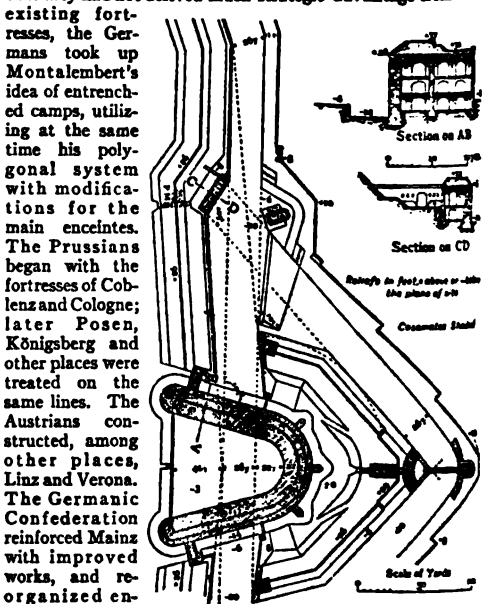
FIG. 37.—Front at Posen.
