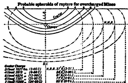
FIG. 73.—Mines.
