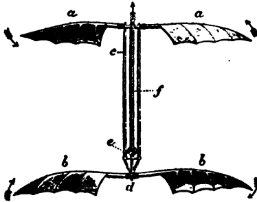
FIG. 38.—Hélicoptère or Screw-Model, by Pénau.
