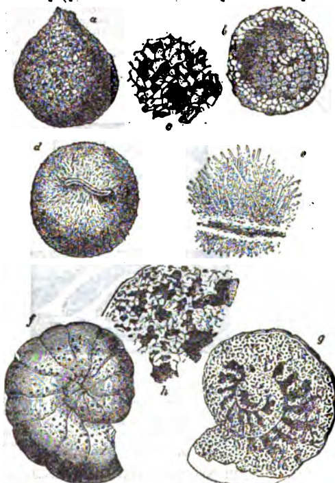
FIG. 19.—Arenaceous Foraminifera.
