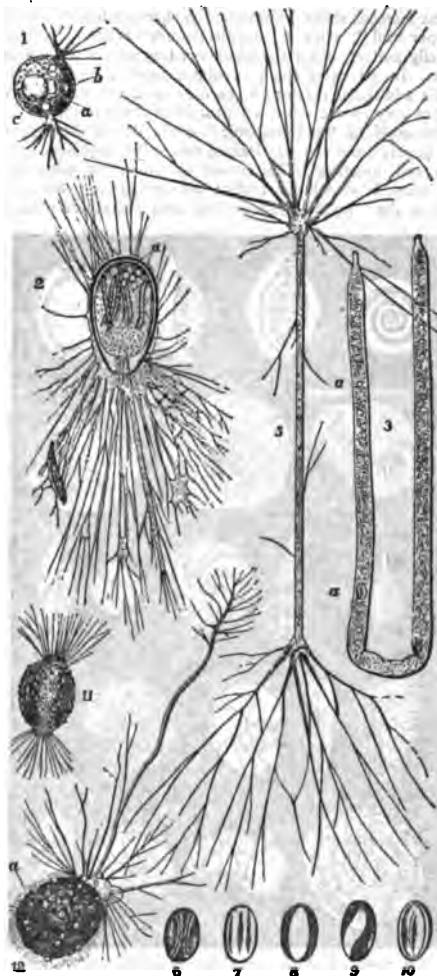
FIG. 2.— Allogromiidea .
