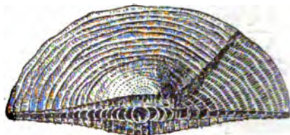
FIG. 15.— Cycloclypeus .
