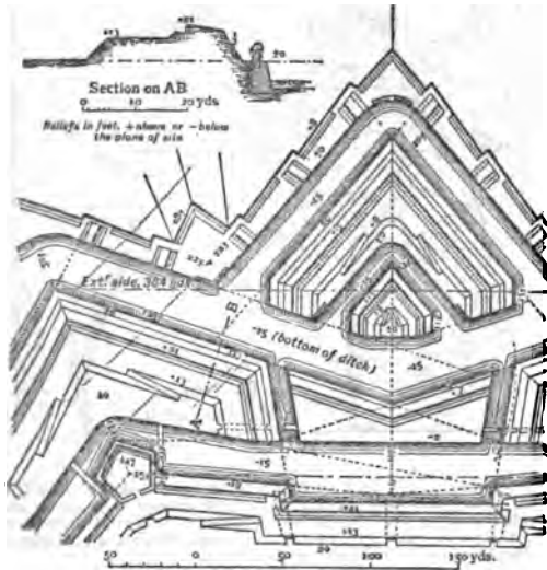
FIG. 26.—Neu-Breisach.
