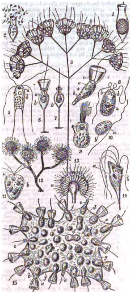
FIG. 2.—Flagellata.
