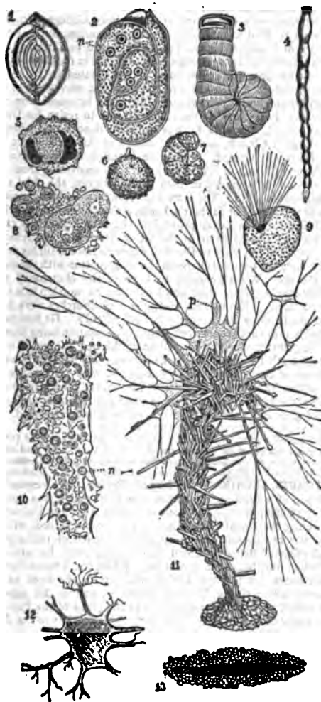
FIG. 22.—Imperforata.
